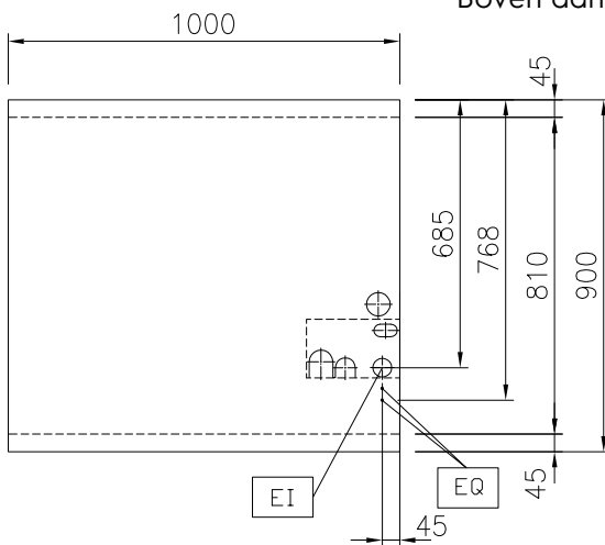
Boven aanzicht
