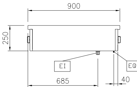
Zij aanzicht
